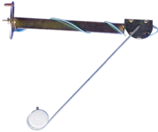
TQ-10 FLOTADOR DE TANQUE UNIVERSAL
