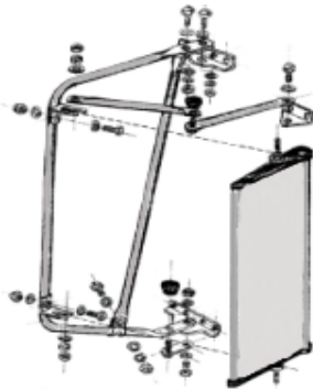
JE-5005 JUEGO DE ESPEJOS DINA 9400/ INTER 9200
